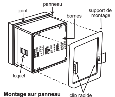
Montage sur panneau
