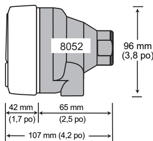
VUE LATÉRALE Montage sur site
