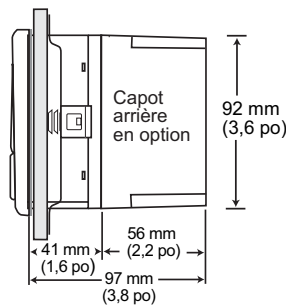
VUE LATÉRALE Montage sur panneau
